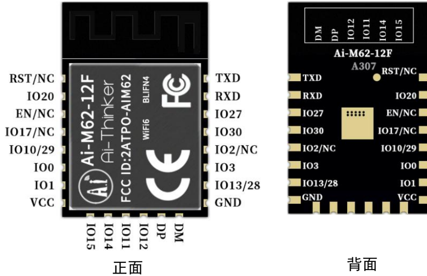
图 6 管脚示意图
